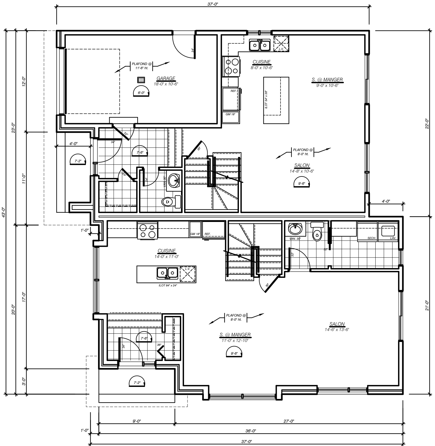
PLAN DU REZ DE CHAUSSEE
