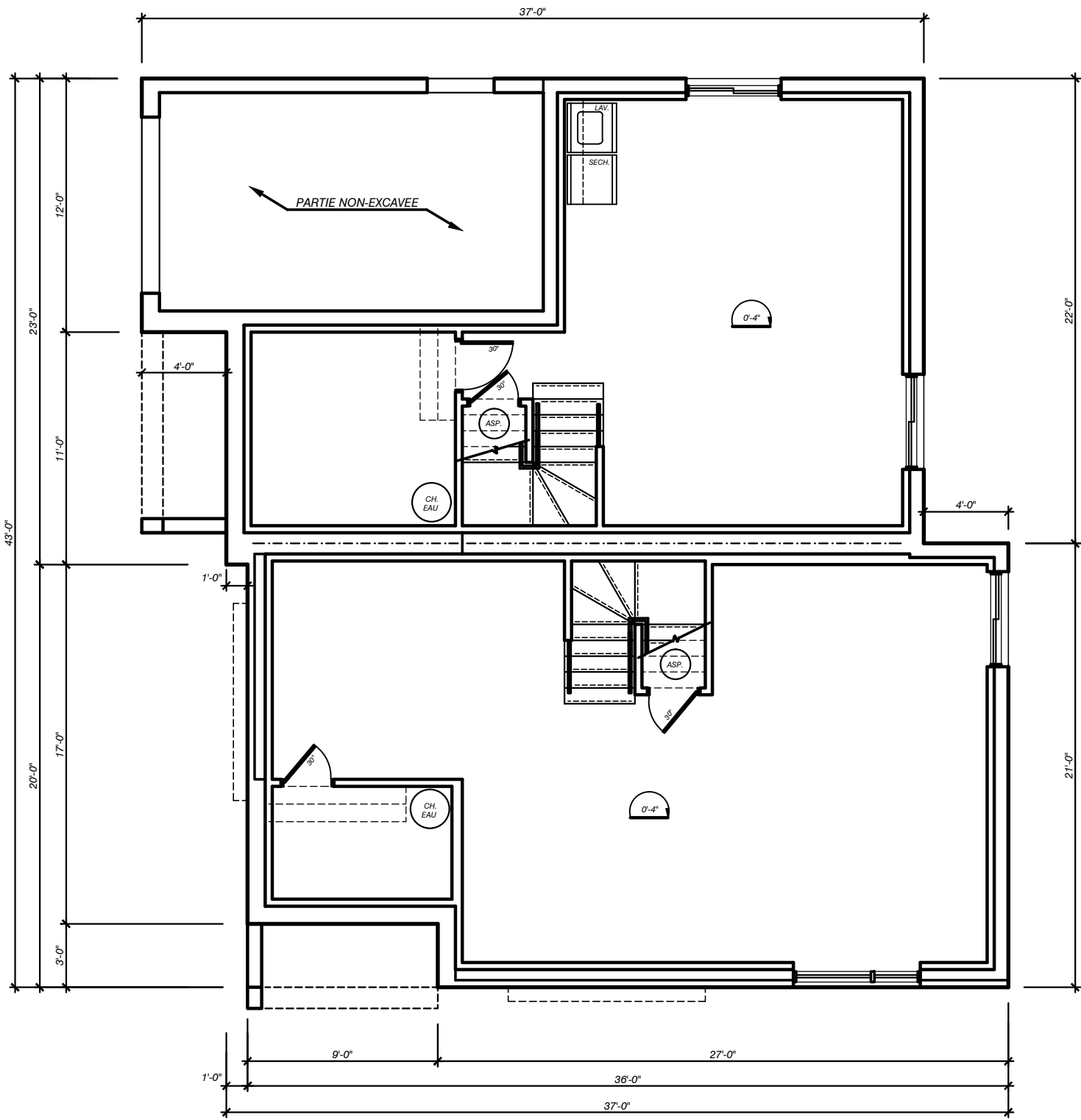
PLAN DES FONDATIONS
